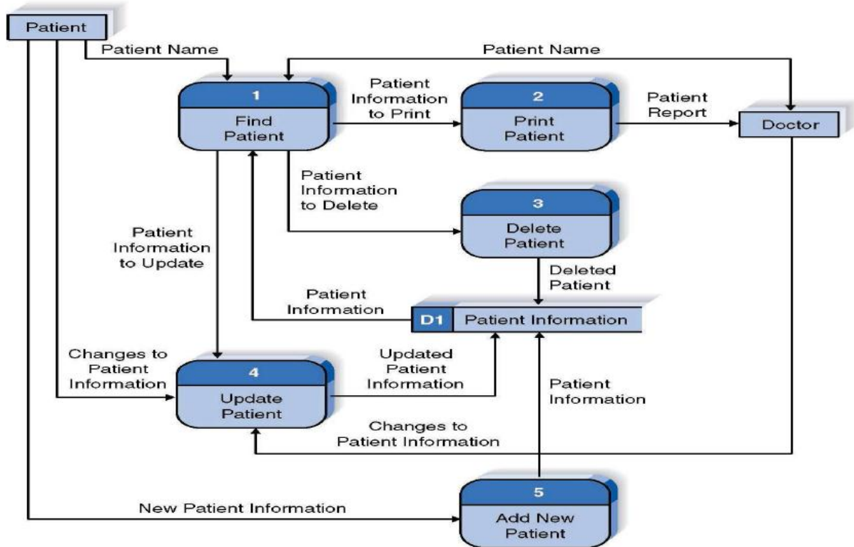
DFD سطح صفر
